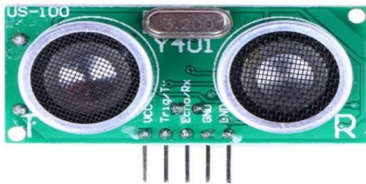
Fig 3.3.- Ultrasonic Sensor
