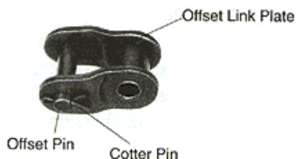
Fig.1.3 :-Offset link
